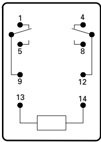
Schaltbild
